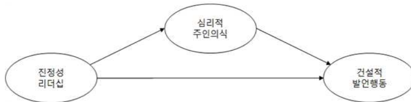
그림 1. 연구모형
