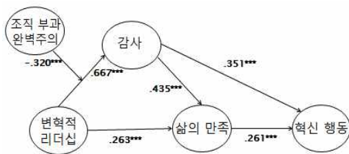
그림 4. 변혁적 리더십에 대한 연구모형 (경로계수는 표준화 계수, * p < .05 , ** p < .01 , *** p < .001 )
