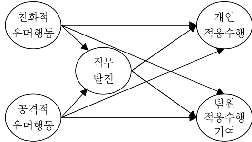
그림 2. 부분매개 모형(경쟁모형)
