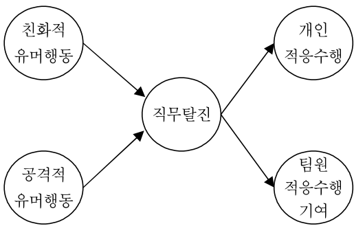
그림 1. 완전매개 모형(연구모형)
